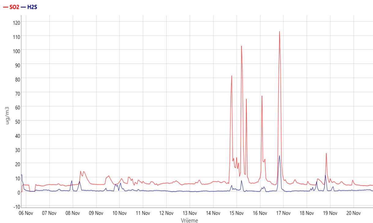
Slika 3. Grafički prikaz rezultata mjerenja plinova \text{H}_2\text{S} i \text{SO}_2
