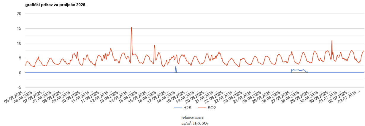
Slika 3. Grafički prikaz rezultata mjerenja plinova H 2 S i SO 2
