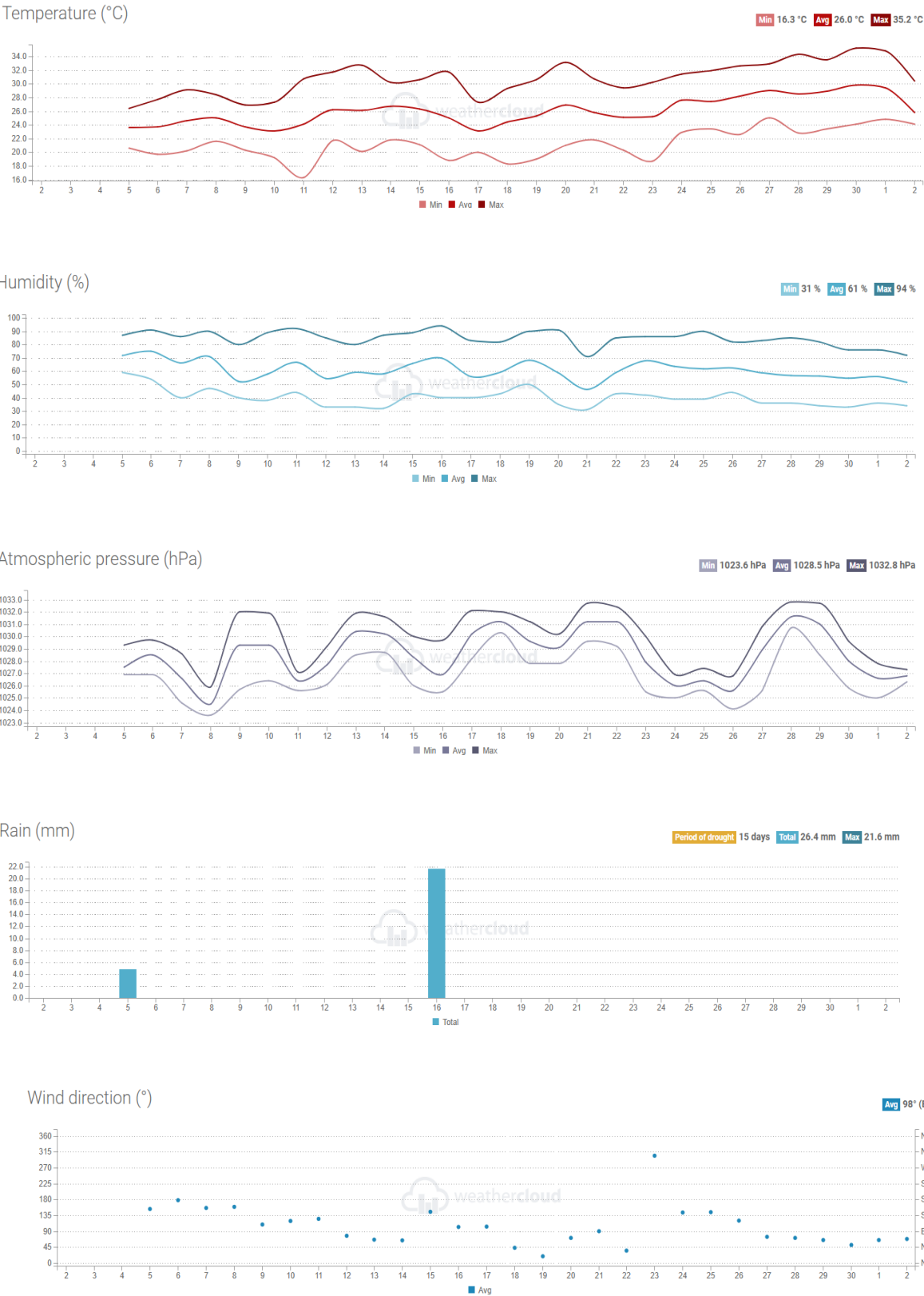
Slika 2. Meteorološki parametri - proljetno razdoblje
